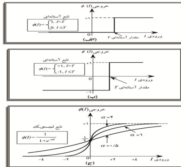
شکل ۷-۳: توابع انتقال برای اعصاب: (الف) تابع فعالسازی آستانه‌ای (وقتی T=0 تبدیل به یک تابع فعالسازی صفر و یک خواهد شد). (ب) تابع فعالسازی علامت (که گاه تابع اندازه‌گیری نامیده می‌شود). (ج) توابع فعالسازی لجستیک برای مقادیر \alpha = 0.5 و \alpha = 1 و \alpha = 2 .
